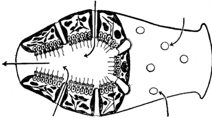
Schema van een klein deel van een eenvoudige spons, waarvan van een stuk is uitgesneden. De pijlen duiden de richting aan van de waterstroom. Natuurgrootte : minder dan 1 mm.
