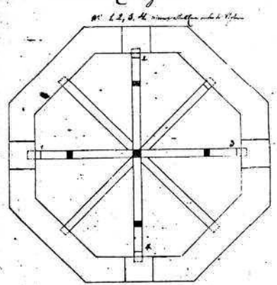
Opmeting van het timmerwerk van de toren, in 1888, door L. Blomme uitgevoerd (Archief Provinciebestuur Antwerpen).
