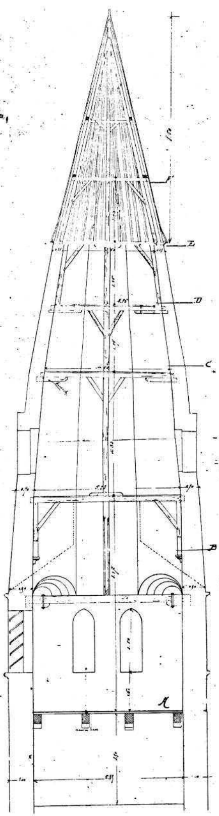
Opmeting van het timmerwerk van de toren, in 1888, door L. Blomme uitgevoerd (Archief Provinciebestuur Antwerpen).
